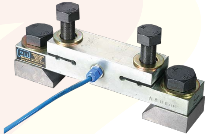
PM30870 LOADCELL
